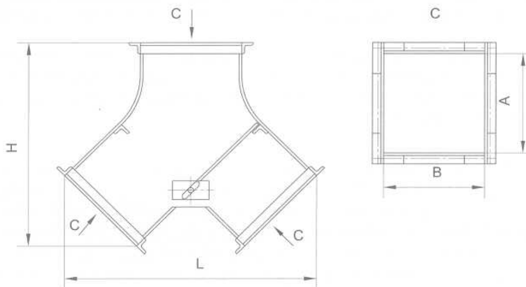
КЛАПАН ПЕРЕКИДНОЙ ВЗРЫВОЗАЩИЩЕННЫЙ Серия 5.904-58
